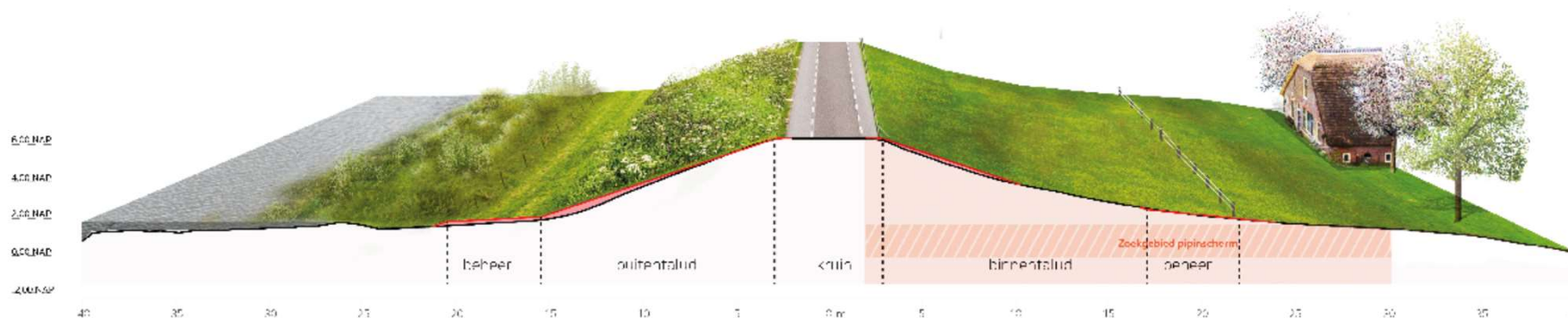
VO profiel t.h.v. DP 125+38
