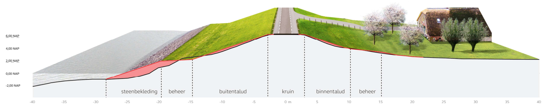
VO profile t.h.v. DP 132+61
