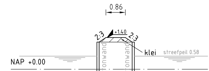
Principeprofiel D kantelstuw schaal 1:100
