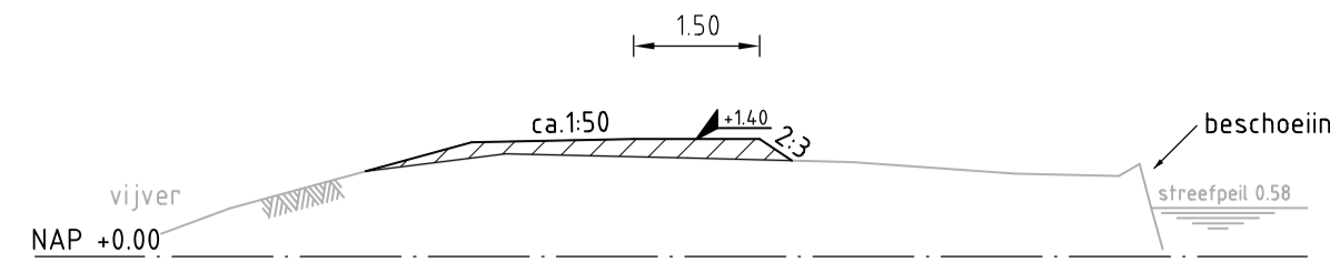
Profiel A schaal 1:100
