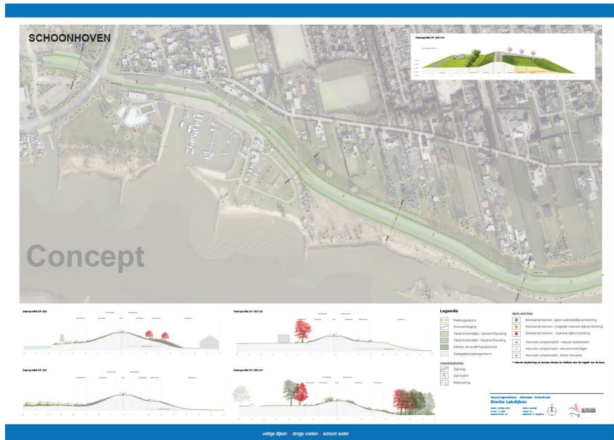
Figuur 1: Tekening Inpassing ontwerp SAS Schoonhoven
