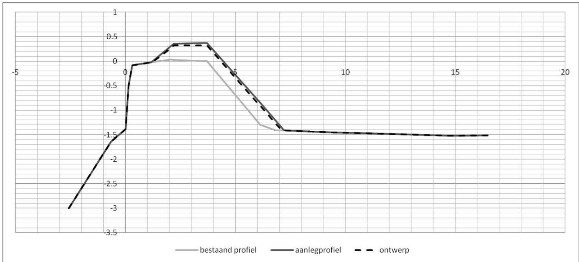
ontwerpprofiel vak 109A3
