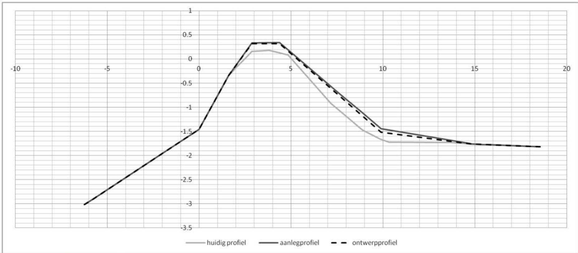
ontwerpprofiel vak 109E
