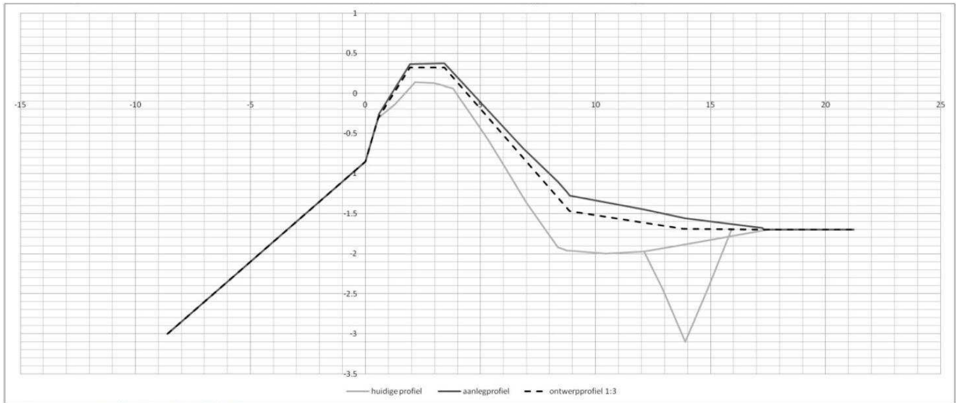
ontwerpprofiel vak 109D
